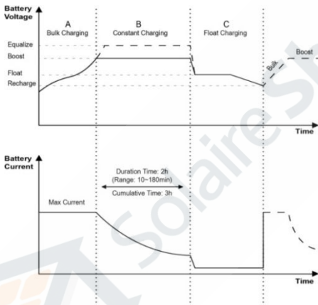
Figure 1-4 Courbe du changement d'étape de la batterie
