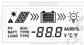
Figure 3-1 ÉcranLCD
