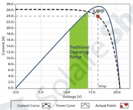
Figure 1-2 Courbe du point de puissance maximale
