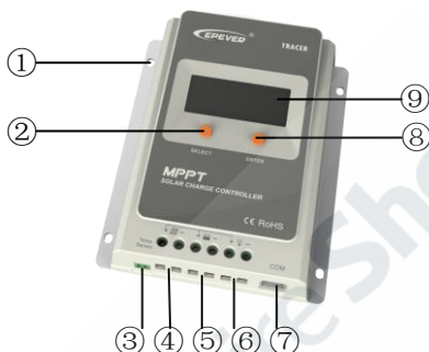
Figure 1-1 Caractéristiques de la gamme Tracer-A
