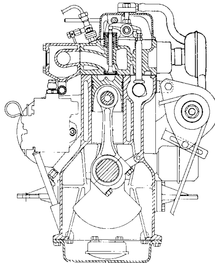
Coupe transversale
