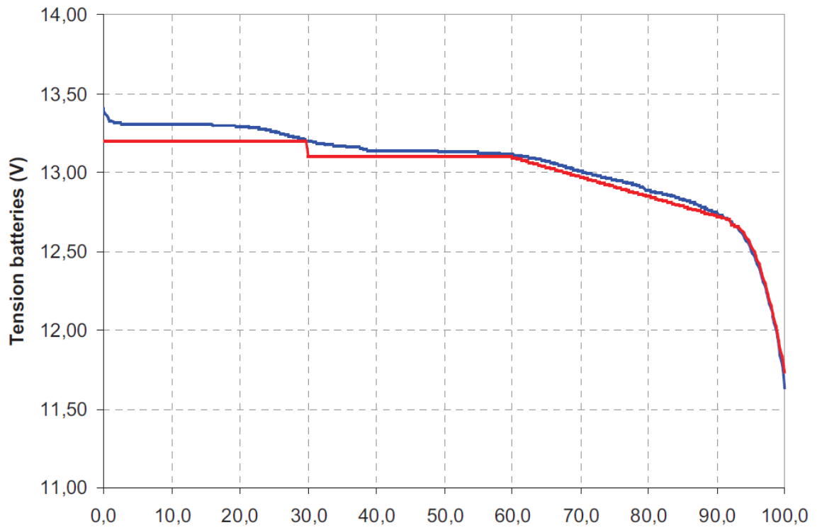
Courbe tension taux de décharge en % des LFP 12V 20Ah
