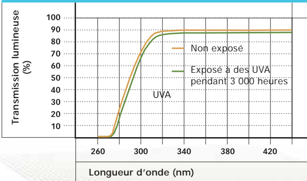
Transmission lumineuse, après exposition de la plaque Altuglas® CN UVD aux rayons UVA
